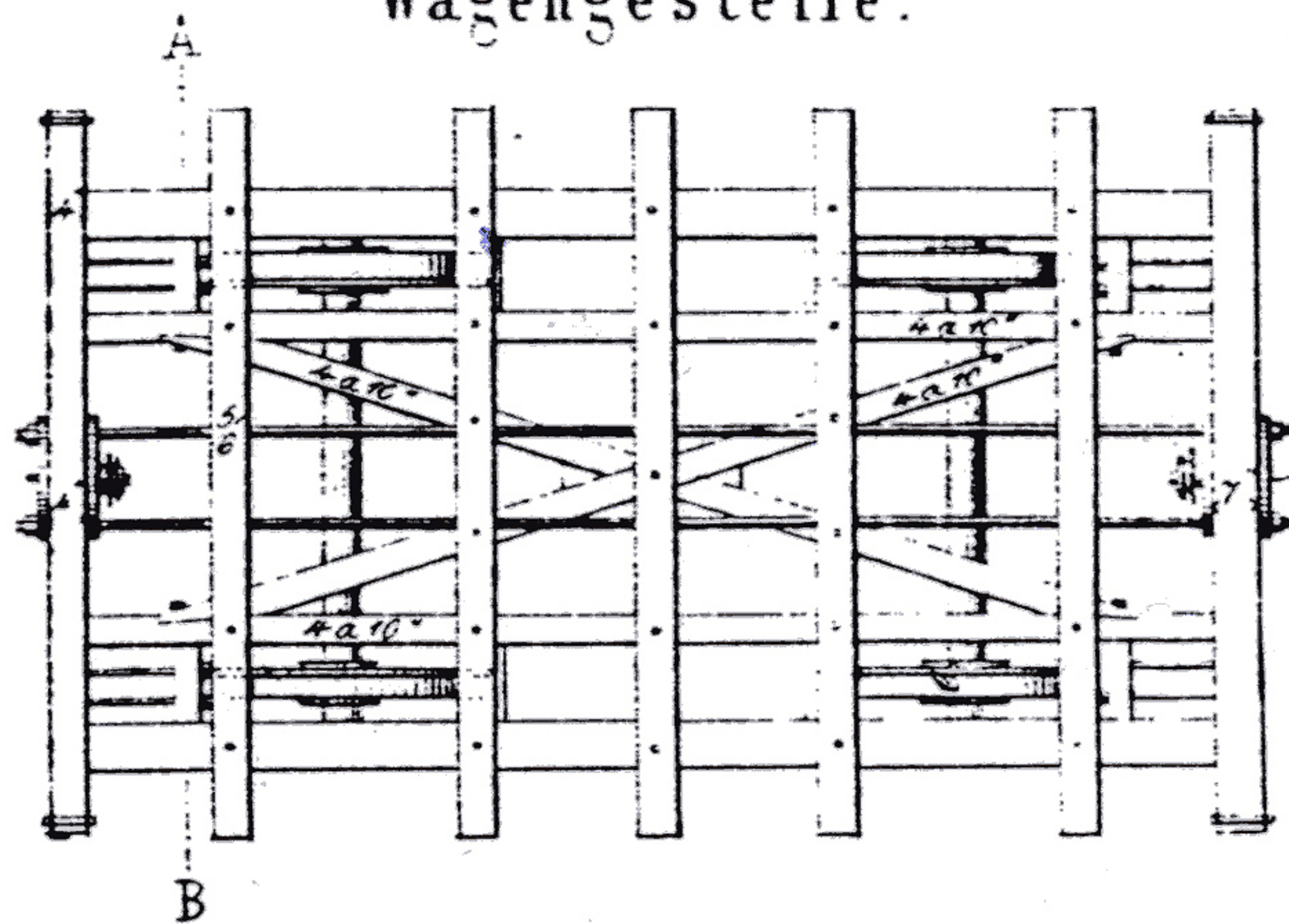
Wagengestelle.
